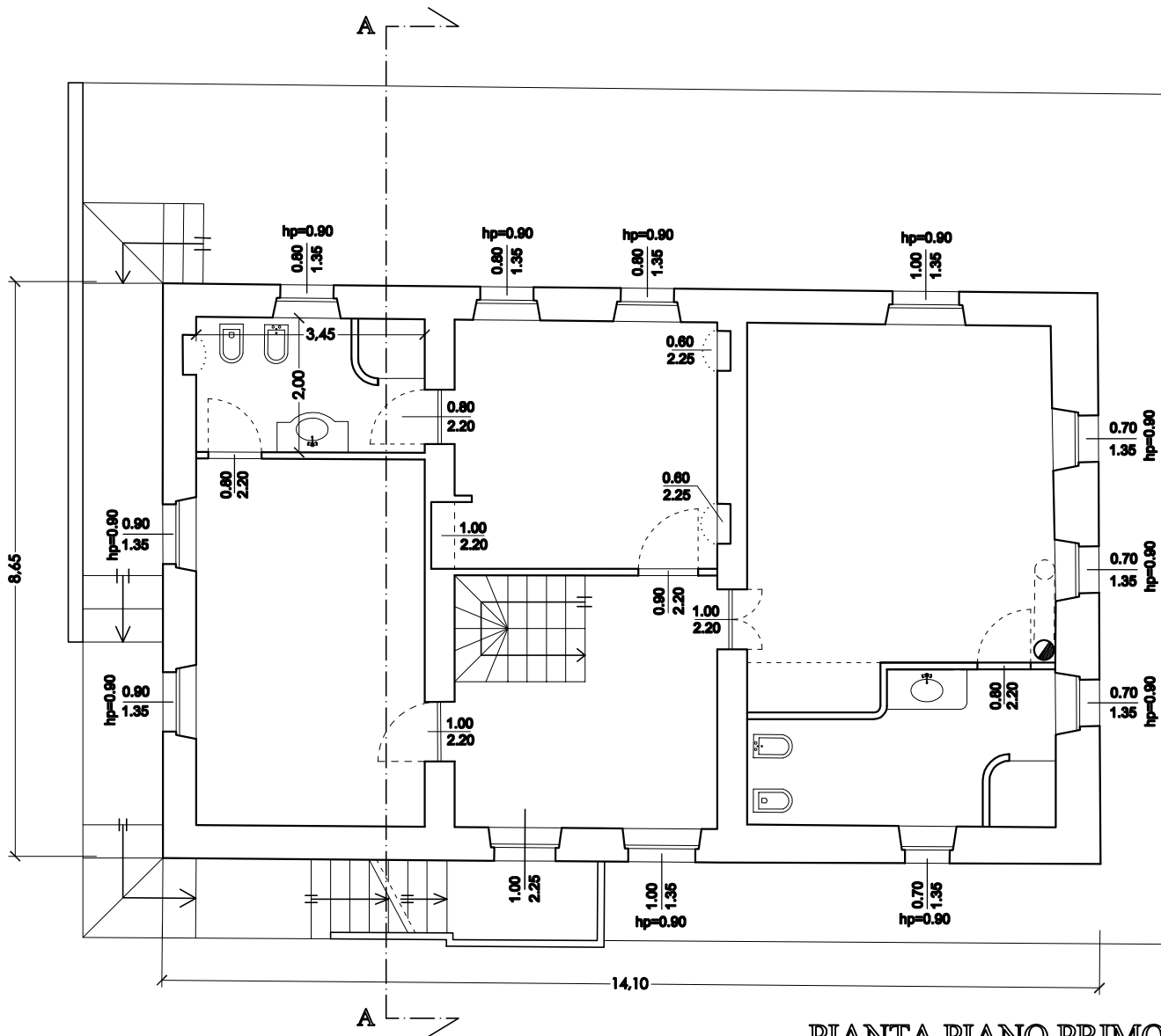
PIANTA PIANO PRIMO pianta aperture scala 1:100
