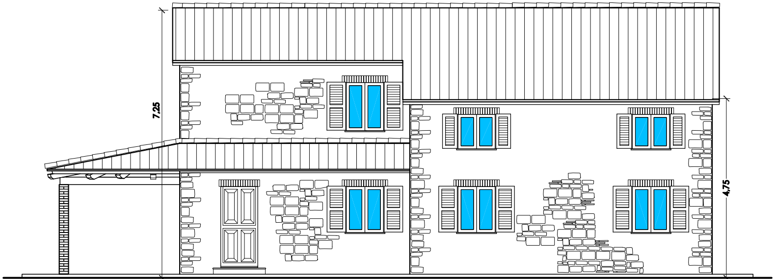
PROSPETTO OVEST
