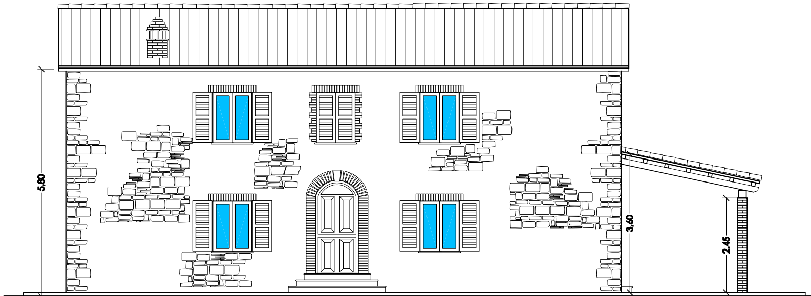
PROSPETTO EST
