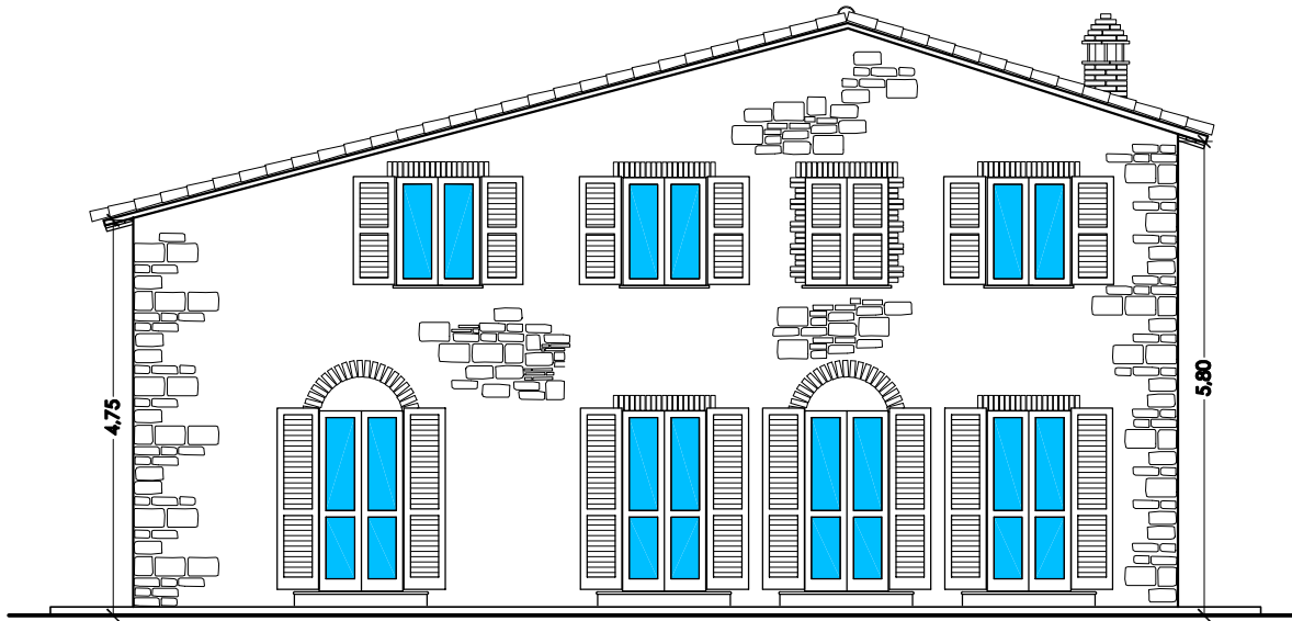
PROSPETTO SUD
