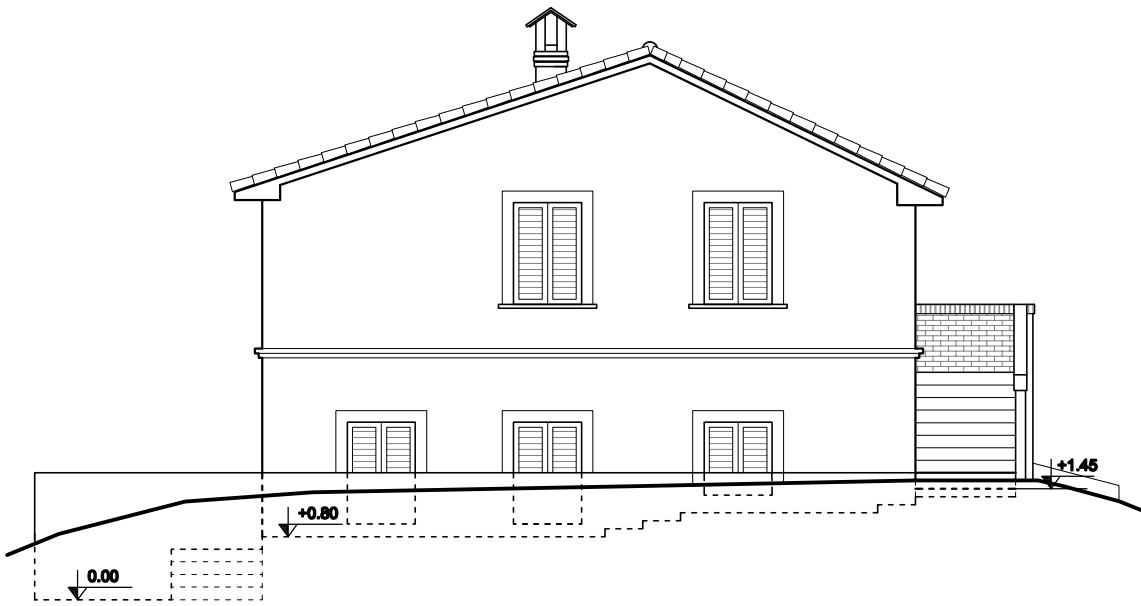
PROSPETTO NORD
