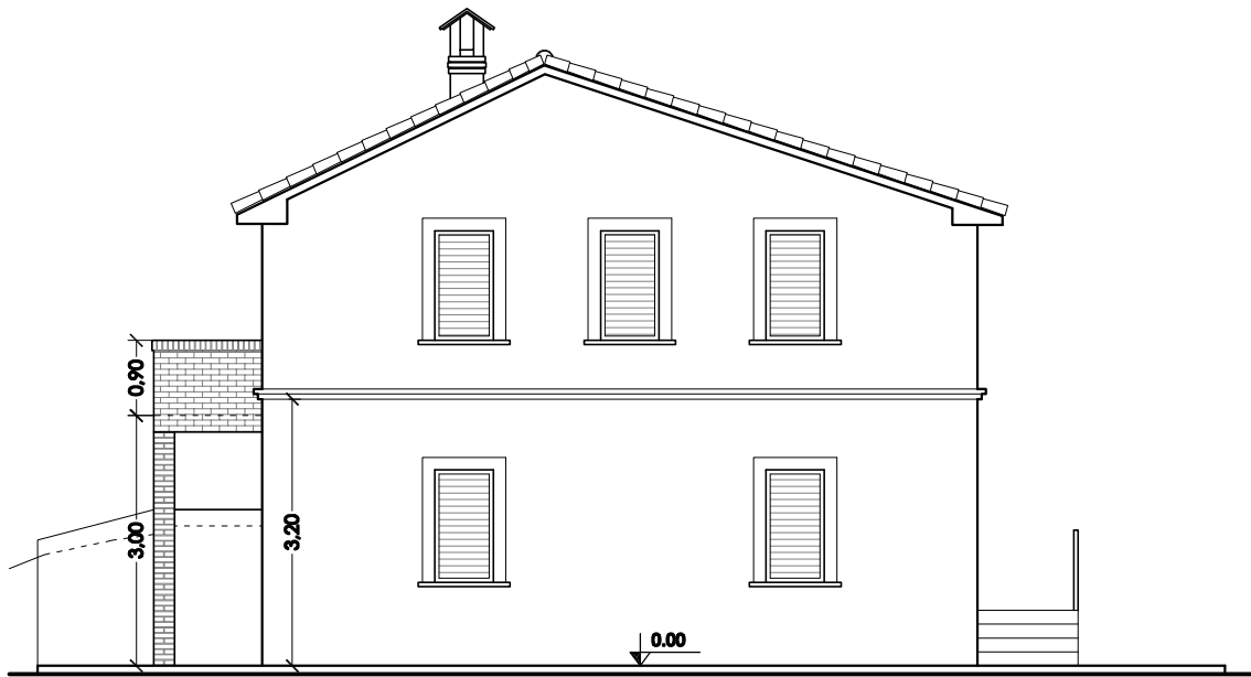
PROSPETTO SUD
